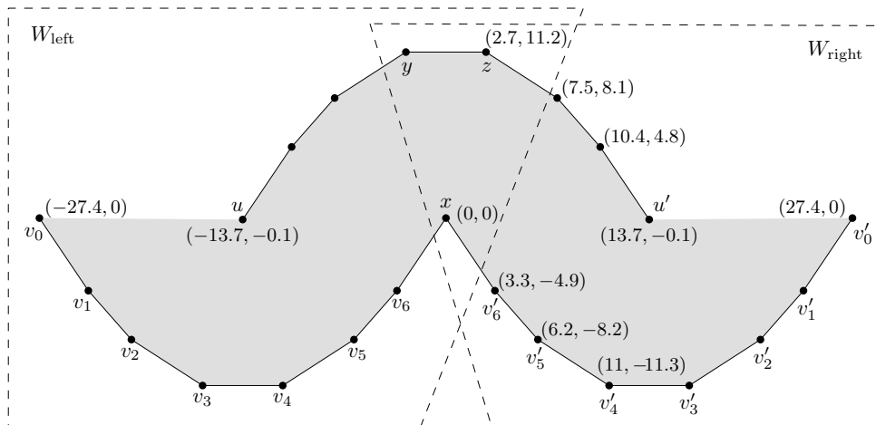
Fig. 9. The point set W in Lemma 5.1
