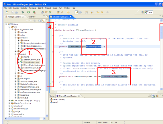
Abbildung 1: Ein Bildschirmfoto von Saros. Die Markierungen zeigen Awareness-Funktionalitäten: 1.) Dateien, welche der Driver gerade bearbeitet 2.) Aktuelle Cursor-Position bzw. Textauswahl des Drivers 3.) Textänderungen des Drivers 4.) Sichtbarer Editierausschnitt des Drivers.
